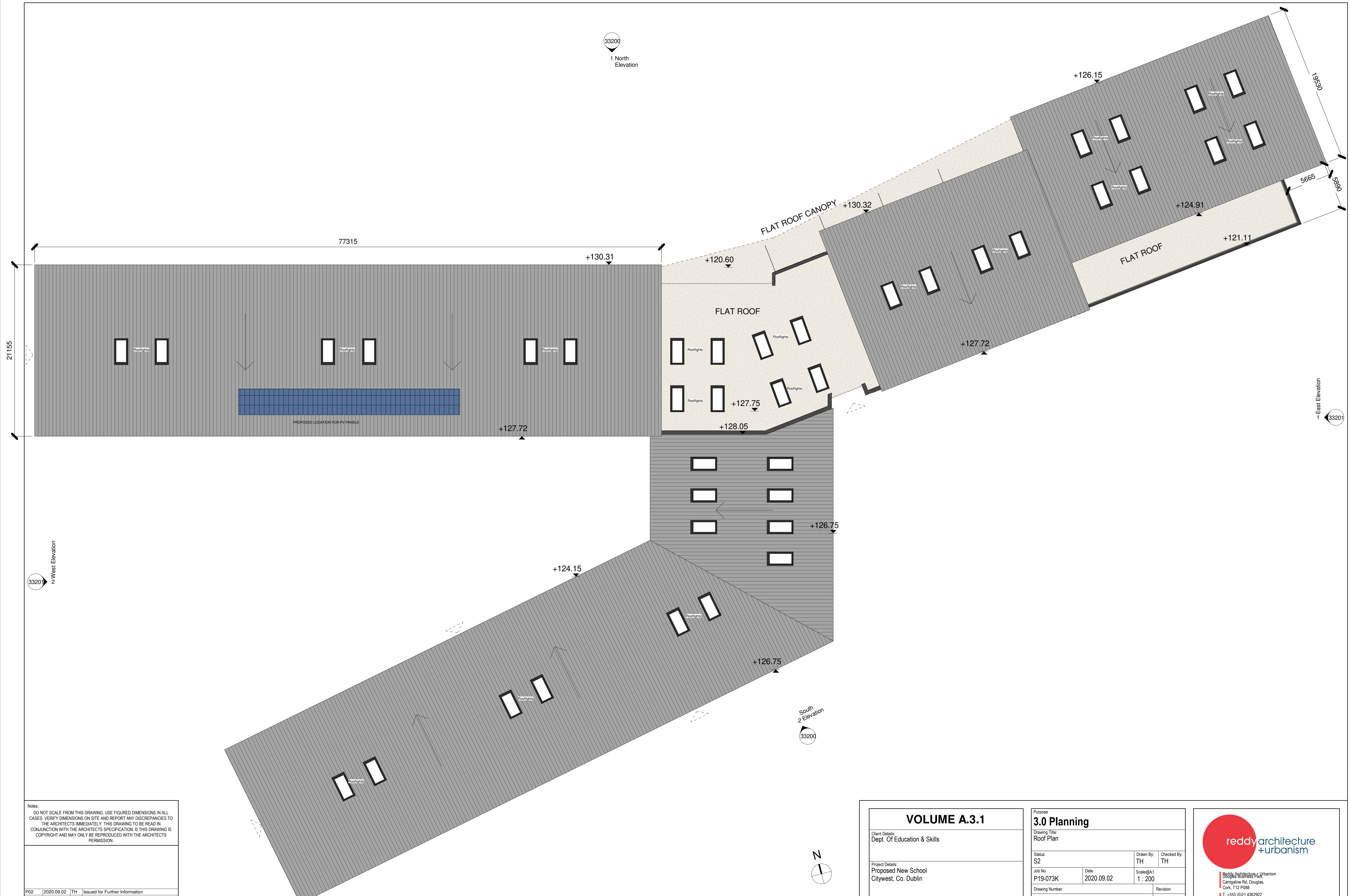
1 Roof Plan 1 : 200
